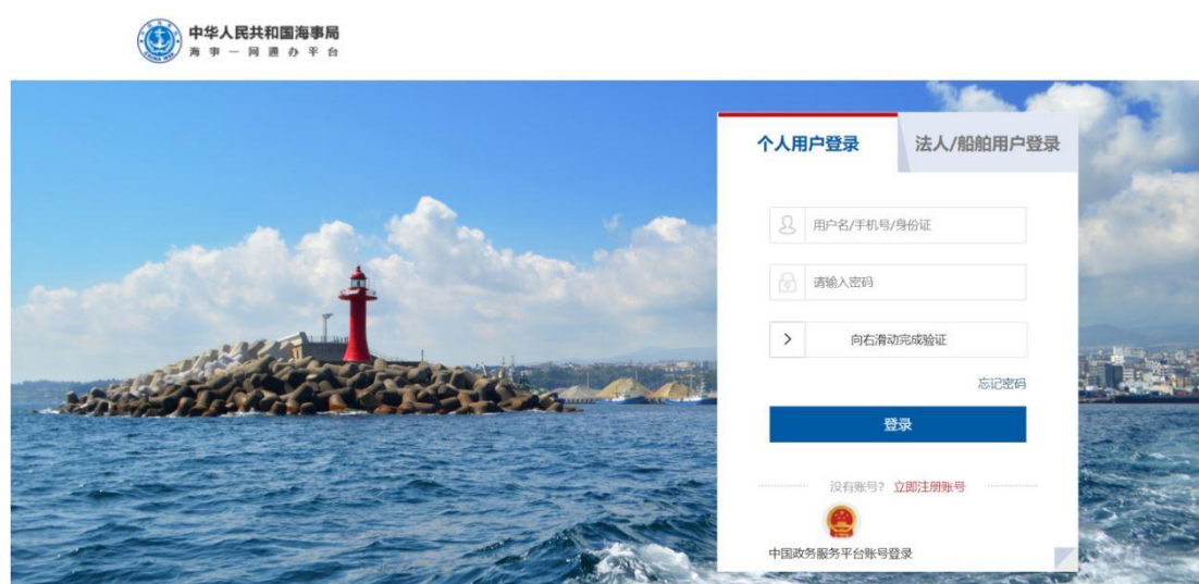
图 1 用户登录
